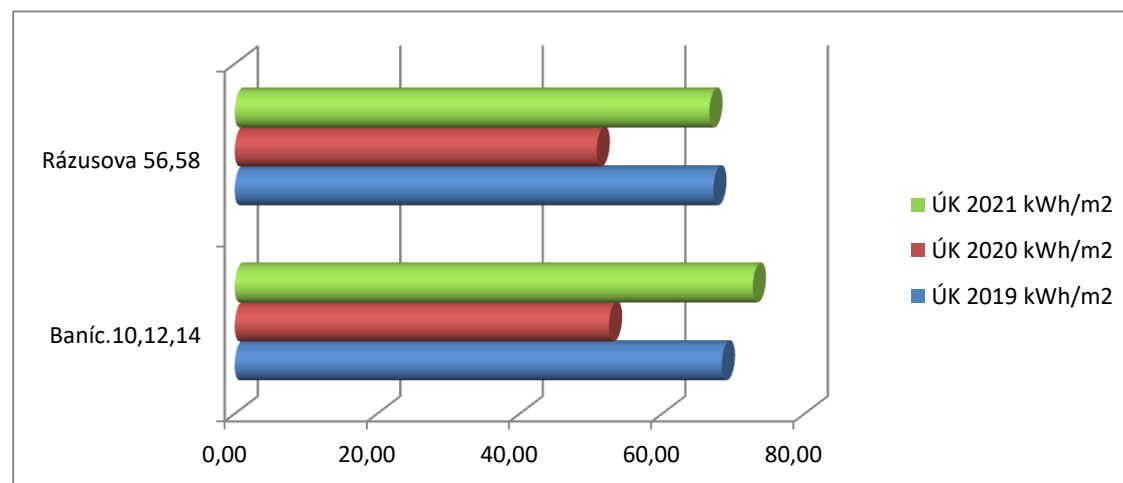
Graf spotreby tepla na ÚK za posledné 3 roky
