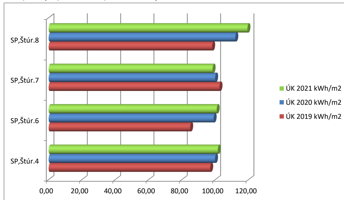
Graf spotreby tepla na ÚK za posledné 3 roky
