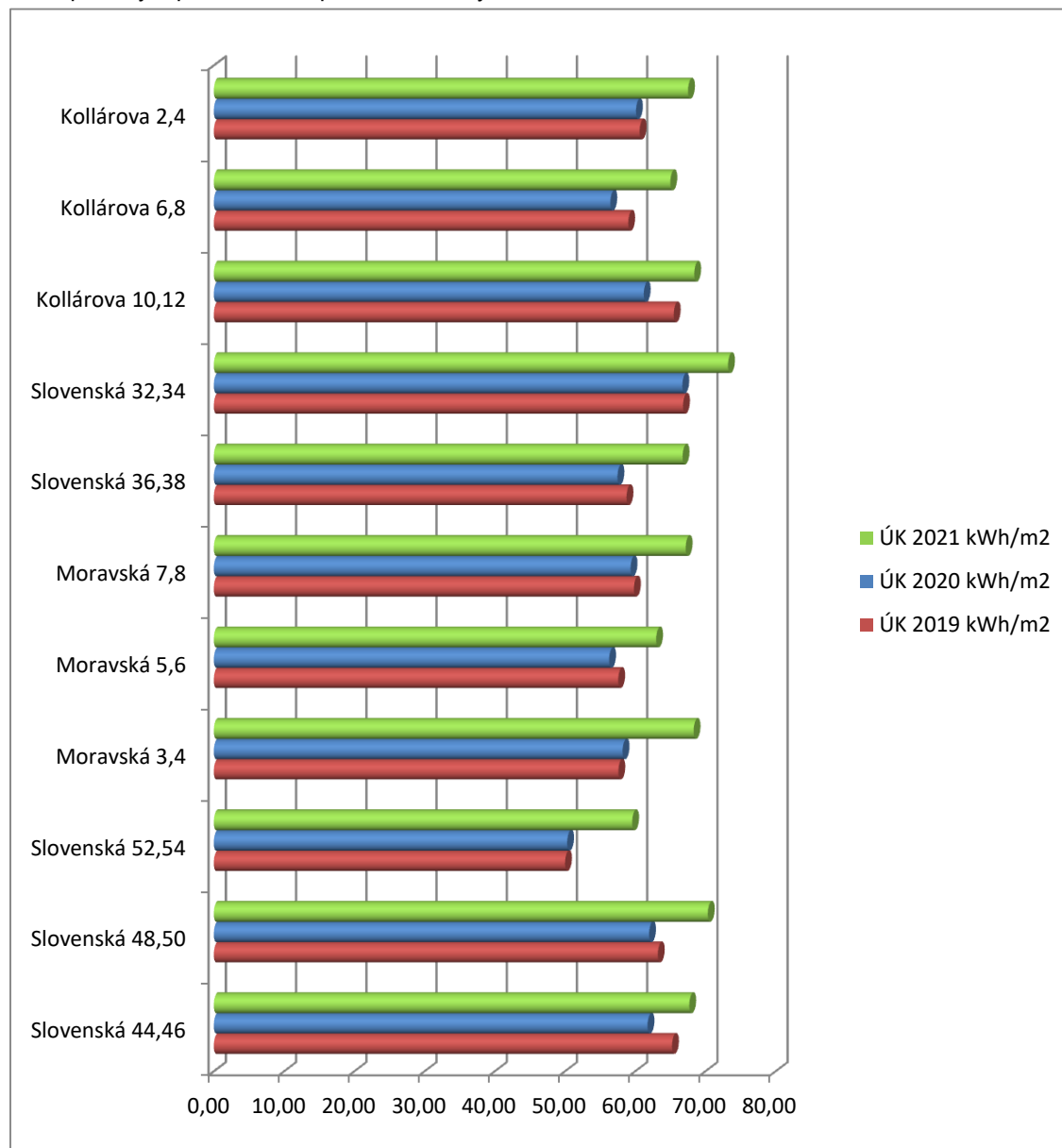
Graf spotreby tepla na ÚK za posledné 3 roky
