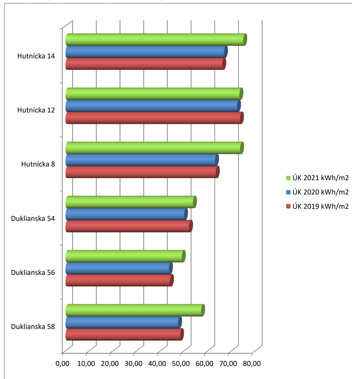
Graf spotreby tepla na ÚK za posledné 3 roky
