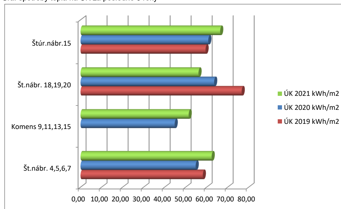
Graf spotreby tepla na ÚK za posledné 3 roky
