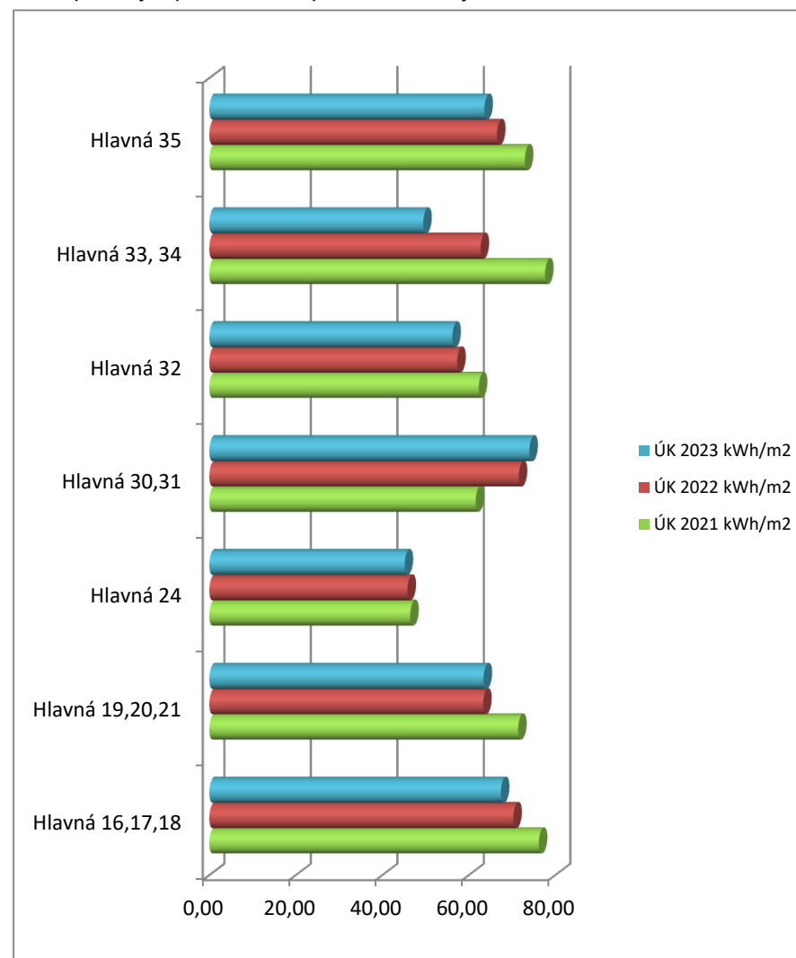
Graf spotreby tepla na ÚK za posledné 3 roky
