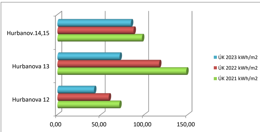
Graf spotreby tepla na ÚK za posledné 3 roky
